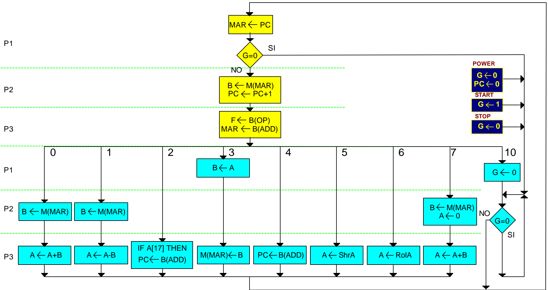
Diagrama de Flujo Computador de Propósitos Generales
